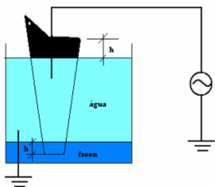
Figura 6. Montagem com manga reta (COPEL, 2007)
